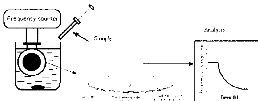
Gambar 1. Skema ilustrasi QCM dengan pelapisan MIP pada elektroda
