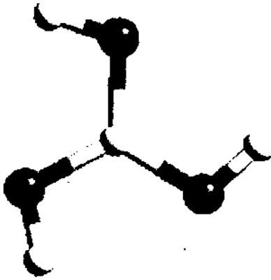
Gambar 4. Proyeksi kerapatan muatan total asam borat
