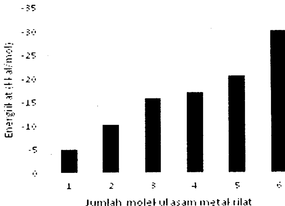
Gambar 5. Histogram energi interaksi satu molekul asam borat dan n molekul asam metakrilat
