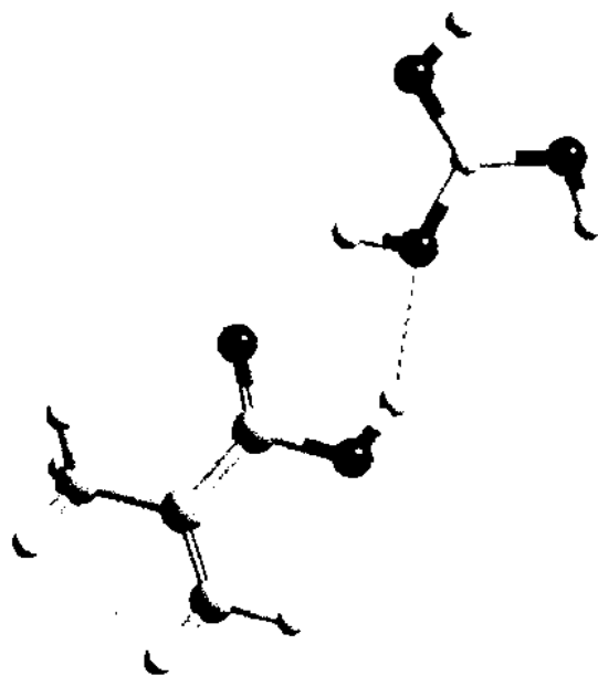
Gambar 6. Ikatan hidrogen yang terbentuk antara molekul asam borat dan asam metakrilat
